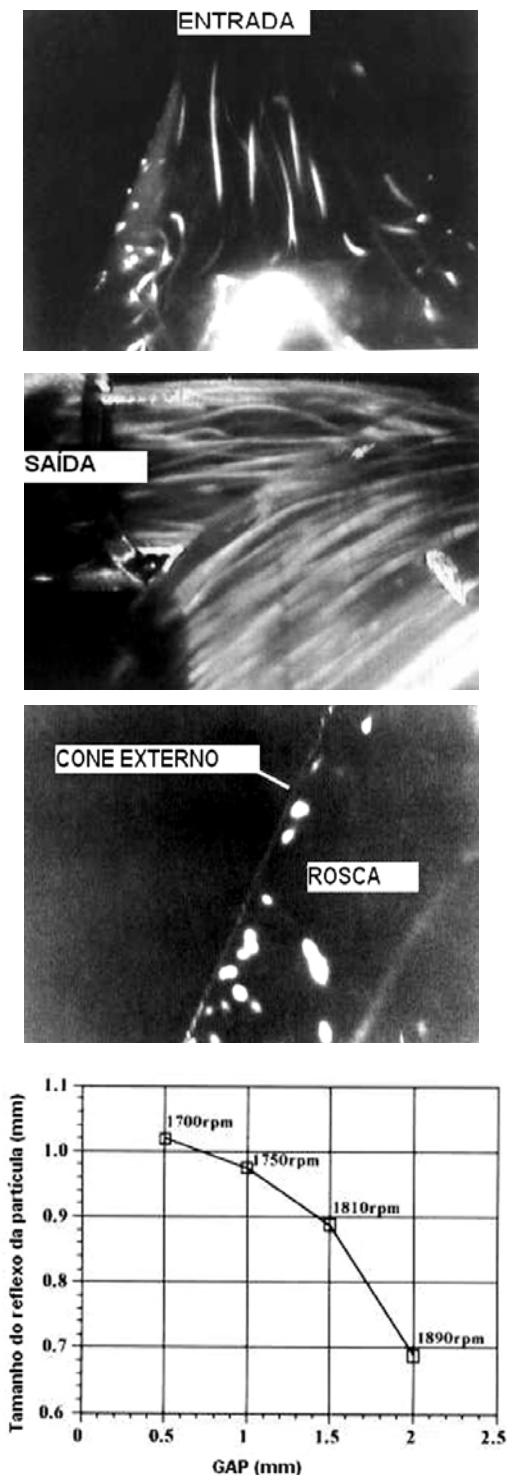
Fig. 7 – Visibilização do Escoamento (“gap” – fenda)
