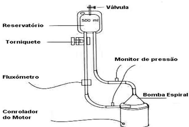
Fig. 3 – Modelo experimental para avaliação da Eficiência Hidrodinâmica
