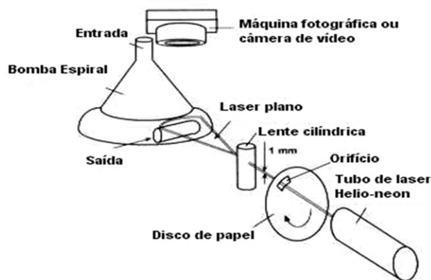
Fig. 4 - Método de Visibilização de Escoamento com laser planar hélio-neon
